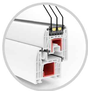
T-Classic Klasyczne dla każdego 7 komór Uw 0,84 W/m 2 K
